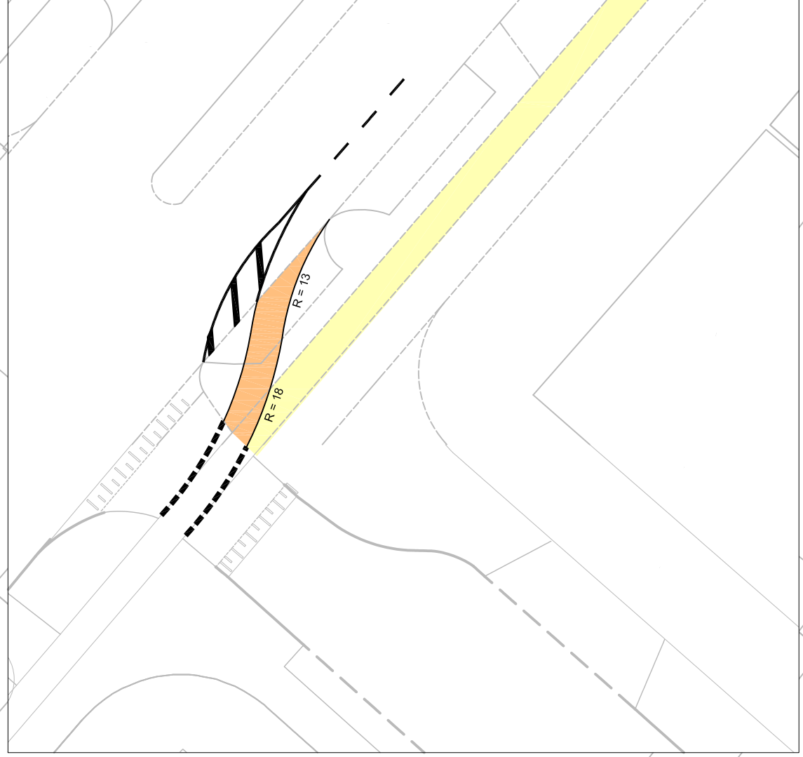
Überleitung Radweg auf Straße nach Einmündung Parkallee / Parkstraße
